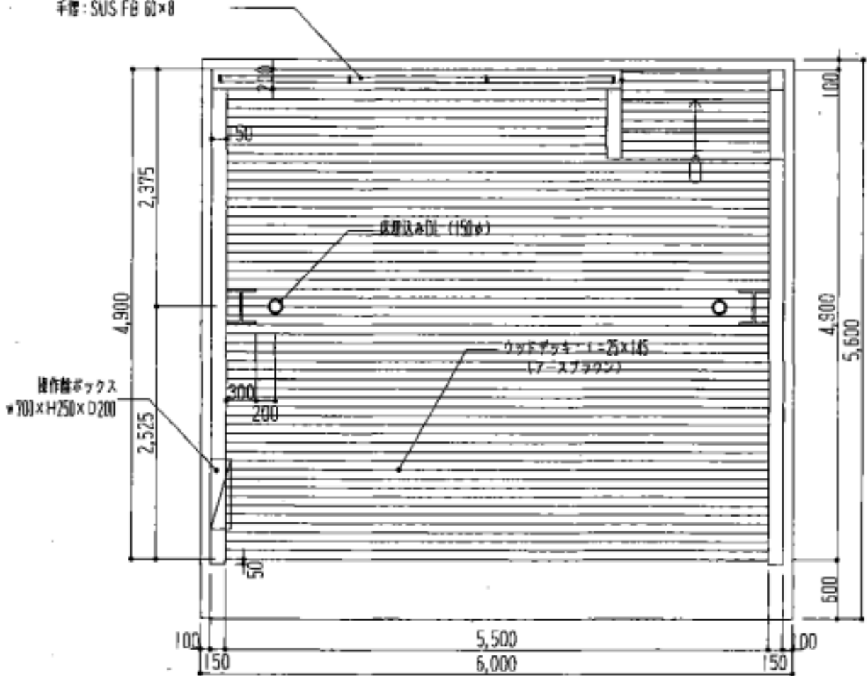
平面図
