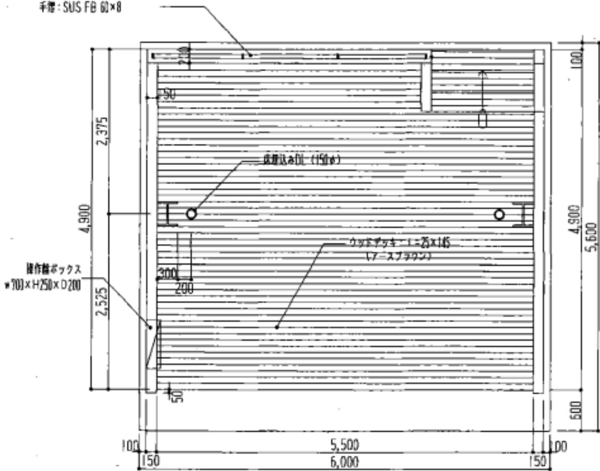
平面図
